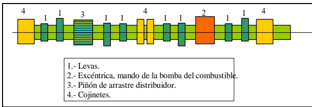
Figura 20.- Árbol de levas
